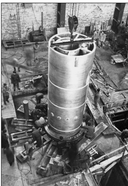
A KFKI épülő atomreaktora (1957)
